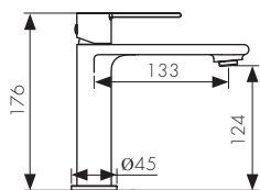
/ Размеры /
