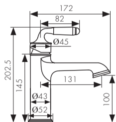
/ Размеры /
