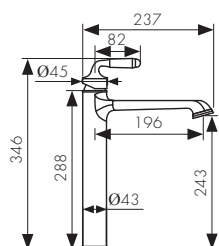
/ Размеры /
